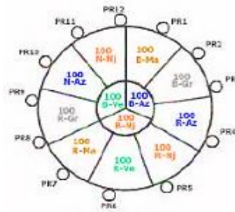
CABLE DE 1200 PARES (12X100)
