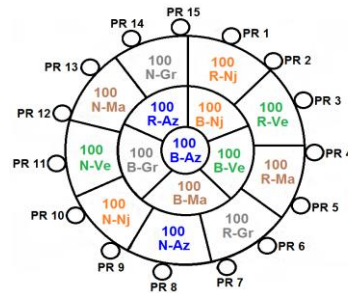
CABLE DE 1.500 PARES (15X100)
