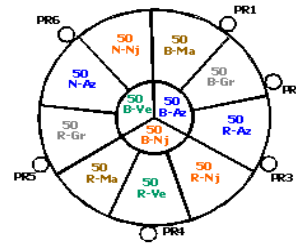
CABLE DE 600 PARES (12X50)
